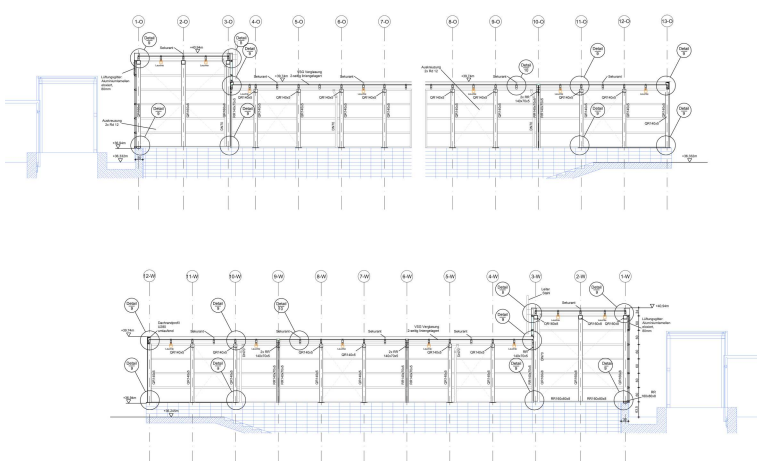
Ausführungsplanung: Schnitte (Zugangsbauwerke Ost und West)
