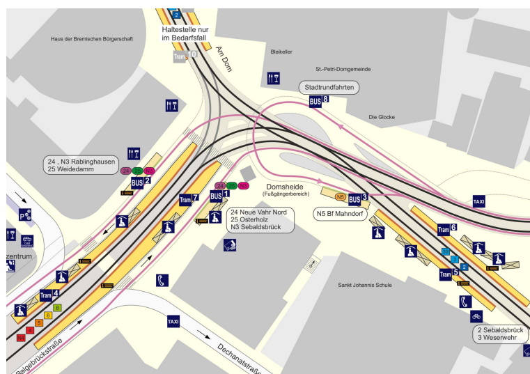
Ebenfalls im Bereich Bremen erhoben: Stationsplan der Tram-Station Domsheide
